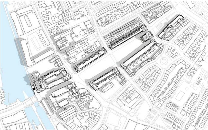
21 juni 09:00
