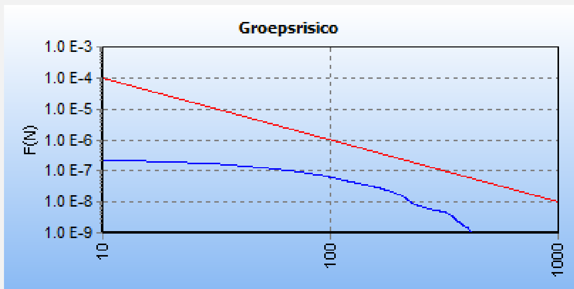
Figuur 6.3 FN curve voor buisleiding W-572-01 van Gasunie voor de kilometer tussen stationing 18930.00 en 19930.00 (bestaande situatie) en stationing 18510.00 en 19510.00 (nieuwe situatie)
